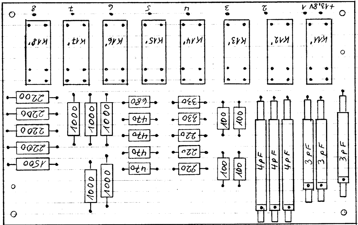
Bestückungsseite der C2-Platine
