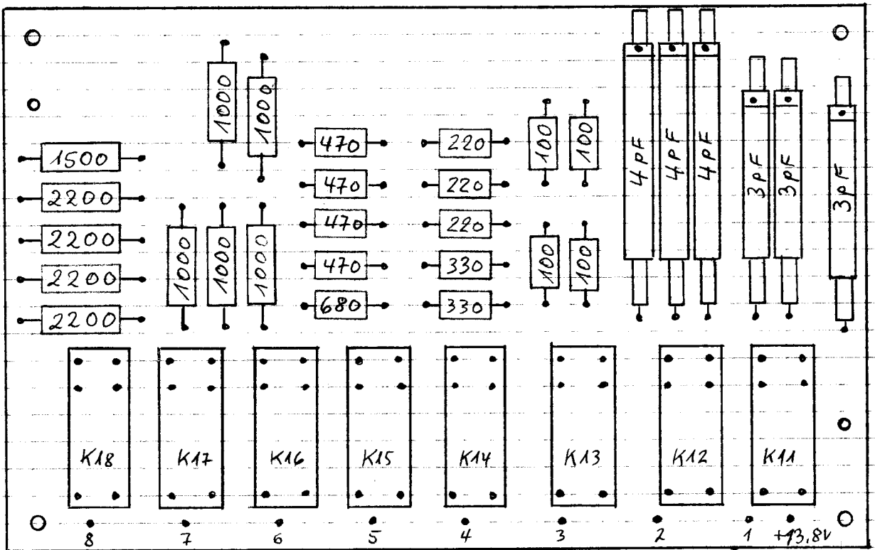
Bestückungsseite der C1-Platine
